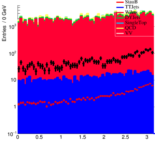
dPhiJMET ZMass cut
