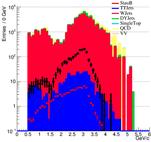
dR_mutau MET > $ 75
