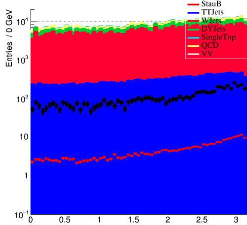
dPhiJMET b-Veto
