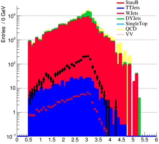
dR_mutau MET > $ 50
