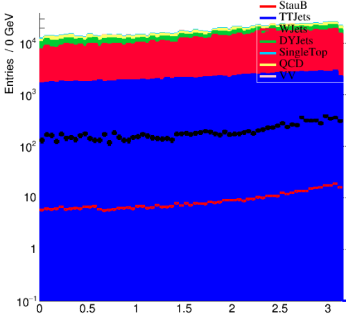
dPhiJMET Jets 3
