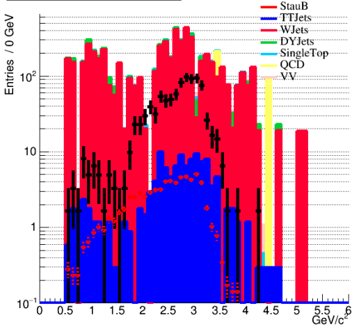
dR_mutau MET > $ 75
