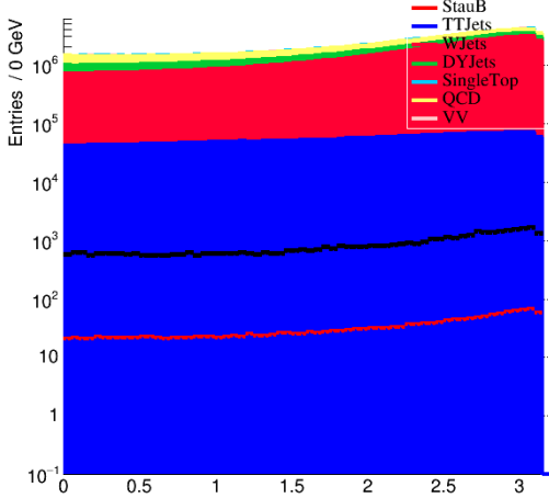
dPhiJMET $DeltaR>0.5$
