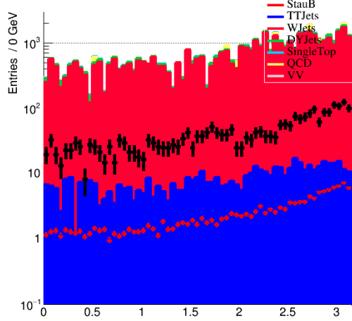
dPhiJMET MET >= 50
